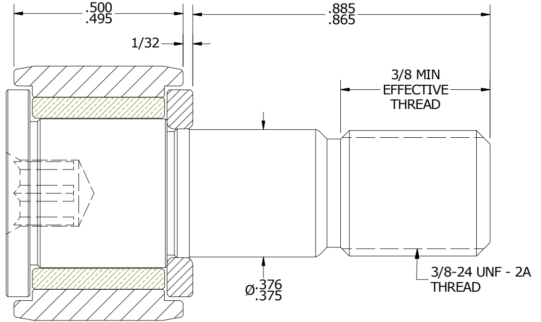
SECTION A-A SCALE 3.500 : 1
