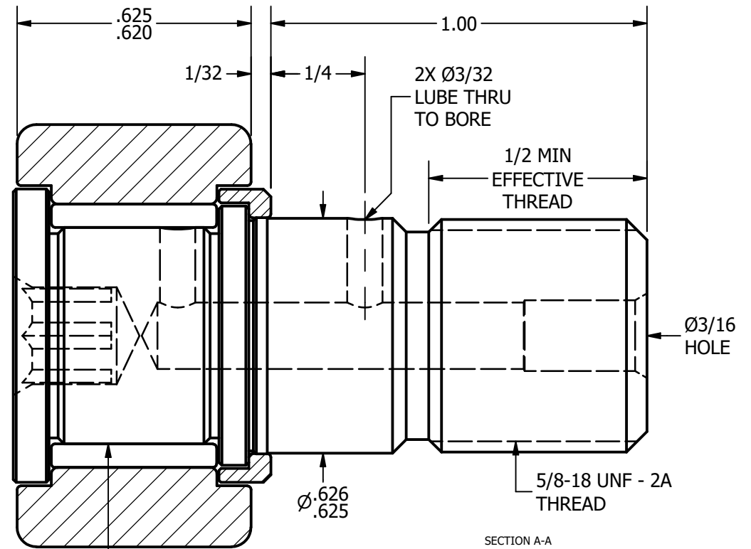
SECTION A-A SCALE 2.75:1
