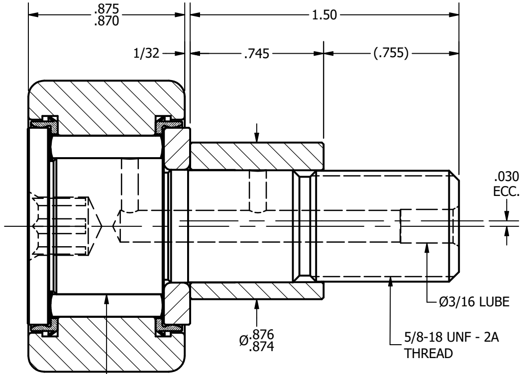
SECTION A-A SCALE 1.875 : 1
