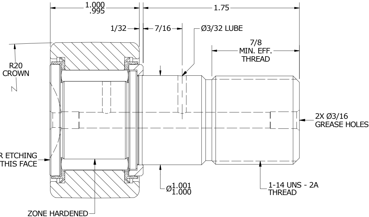
SECTION A-A SCALE 1.625 : 1
