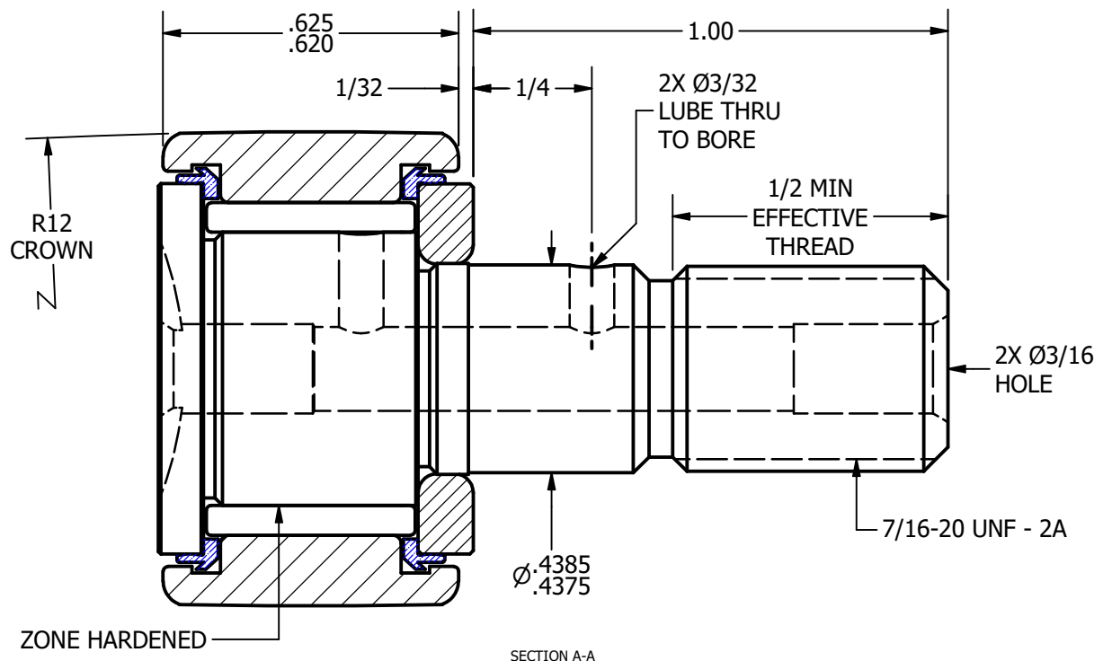
SECTION A-A SCALE 2.75:1
